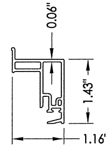
4 LOCK STILE
